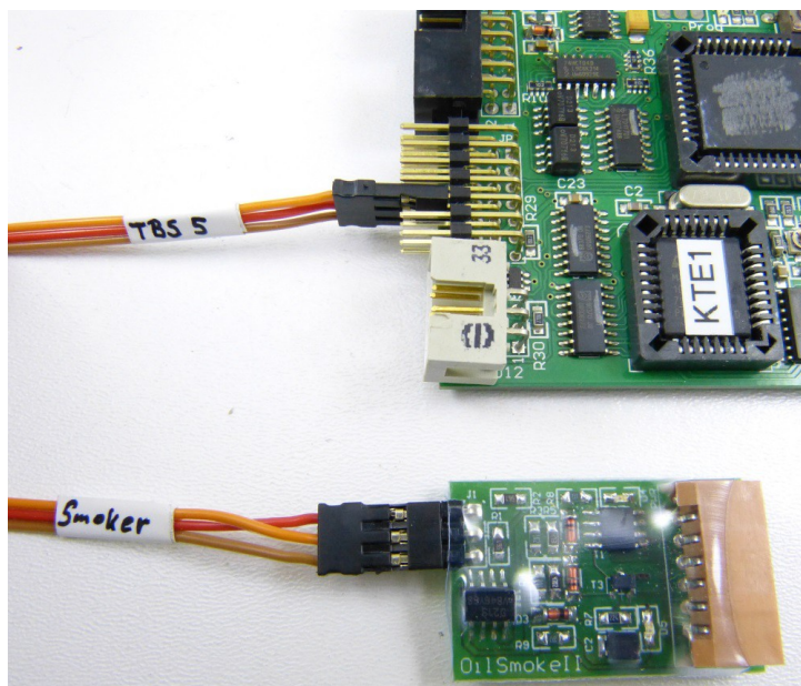
TBS5 Soundmodul (3. Steckplatz von unten)
